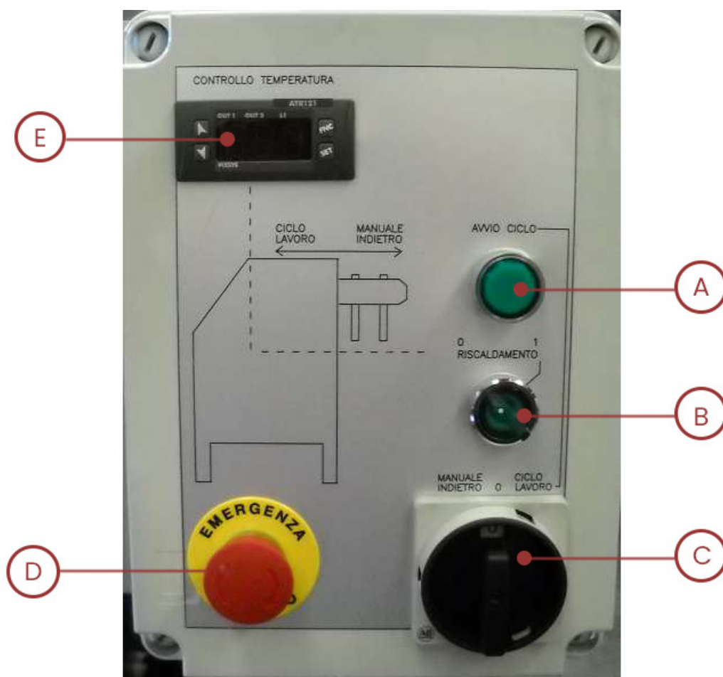
ABB. 1 Bedientafel
