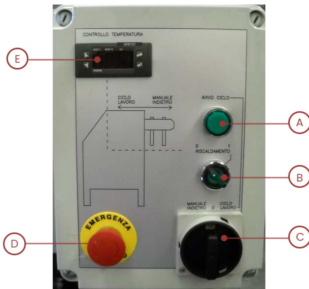
FIG. 1 Quadro comandi
